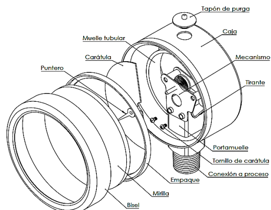
Componentes de un manómetro
